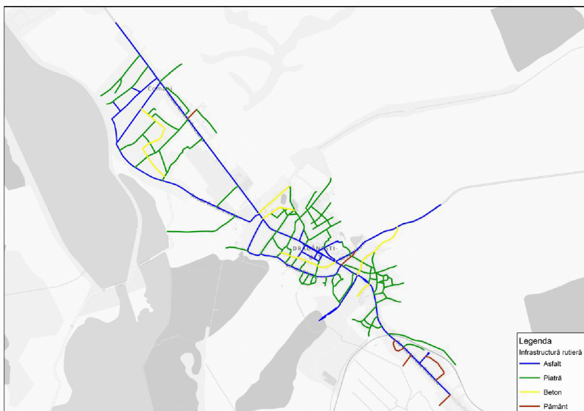
Figura 2.7. Distribuția străzilor în funcție de tipul îmbrăcămînții.
